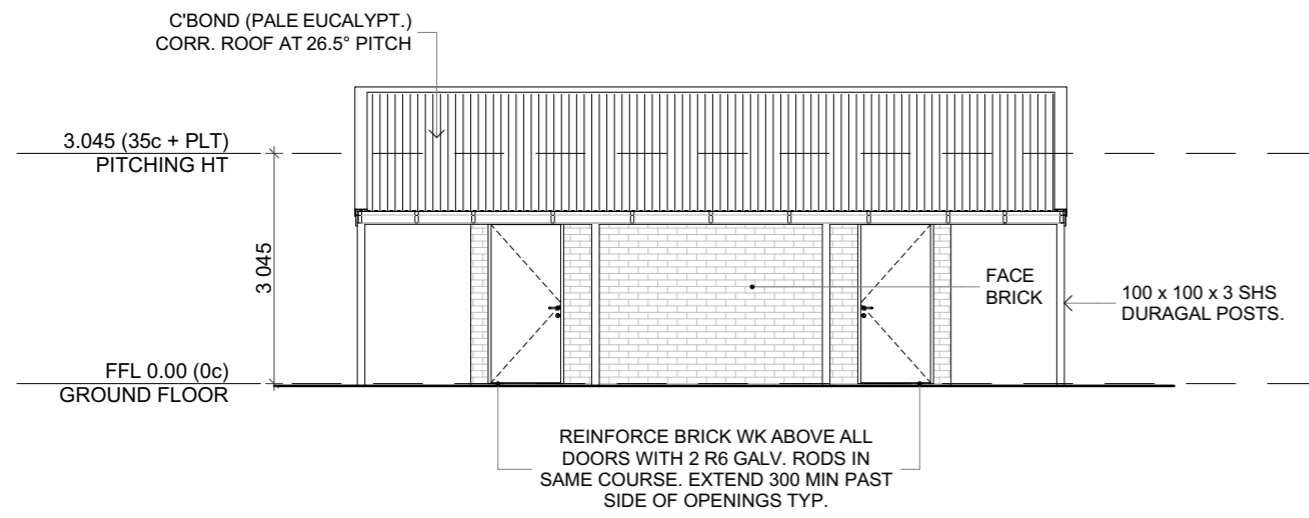
ELEVATION E-1 1:100 A2
