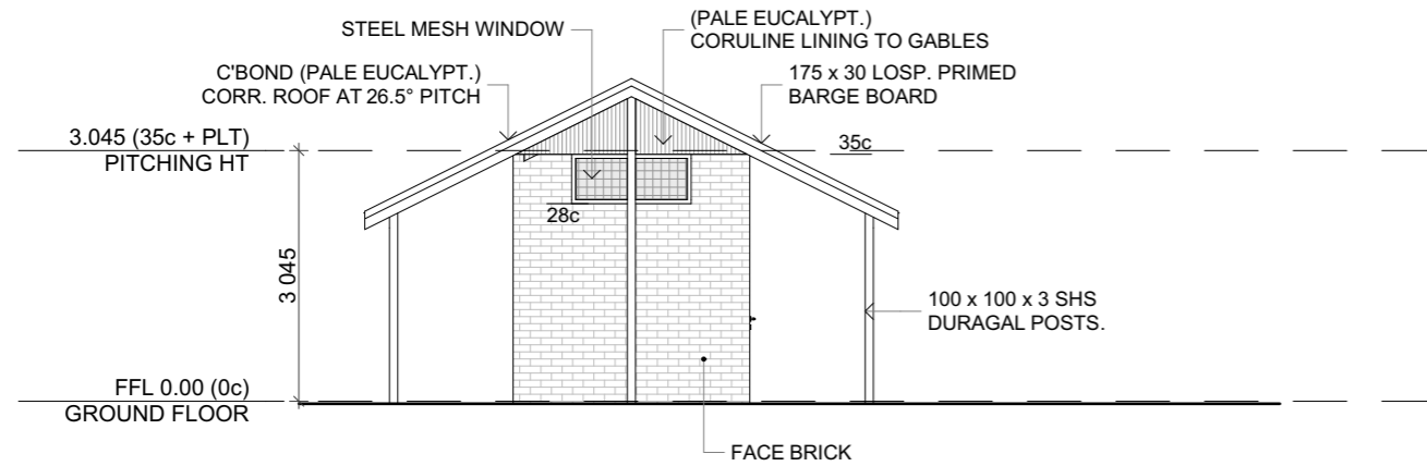
ELEVATION E-4 1:100 A2
