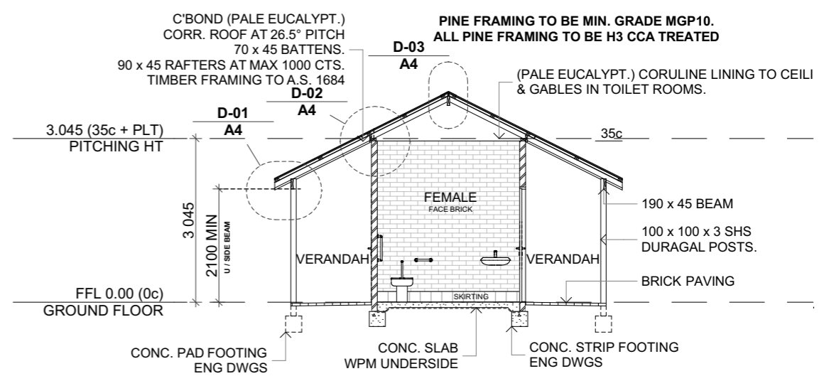
SECTION A:A 1:100 A2
